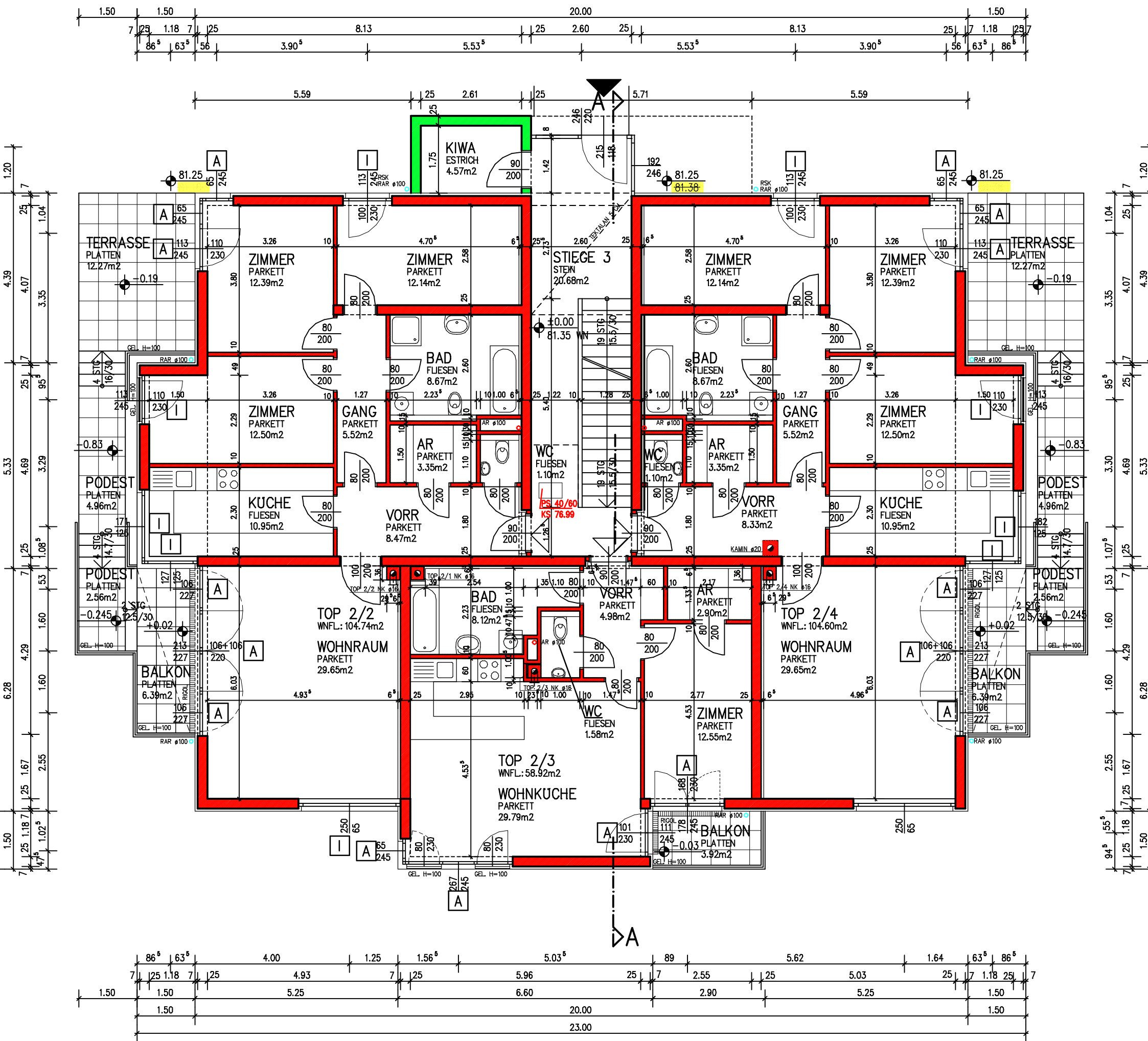
ERDGESCHOSS
