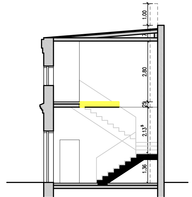
SCHNITT C-C
